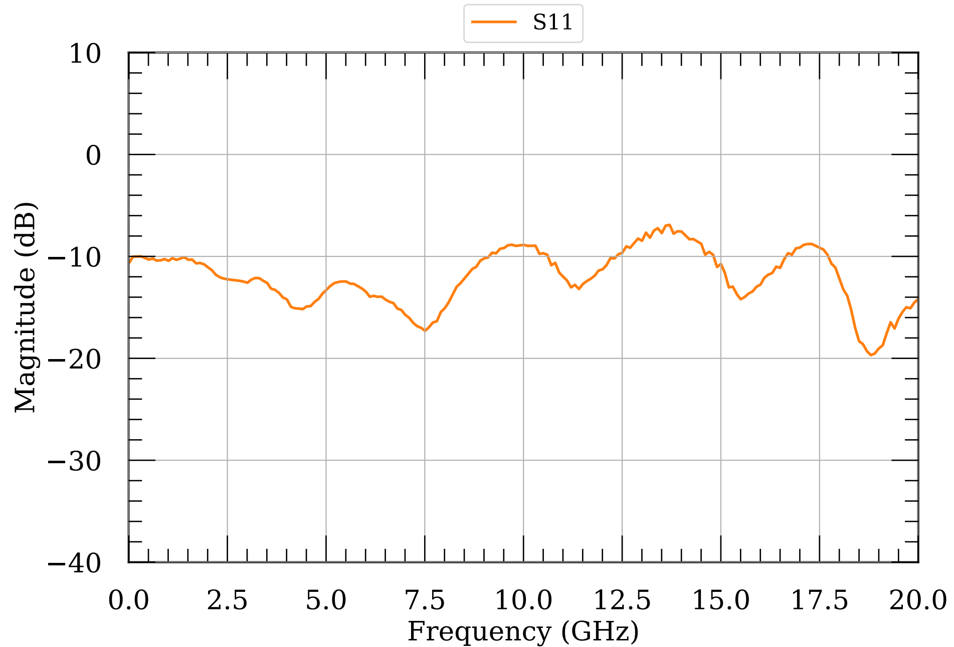
LNA S-params module020v2
